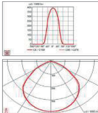
Lichtverteilungsdiagramm
