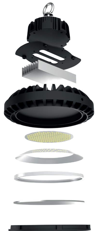
3-D Zeichnung
